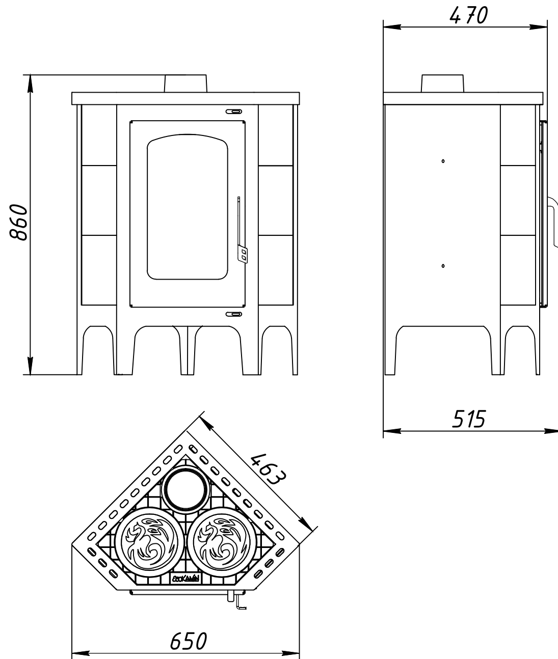
Печь-камин "Бавария" угловая с плитой РК 123, РК 123Н
